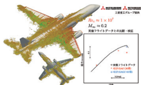
▲図2 FVHC-ACEを用いた三菱重工グループによる民間旅客機LES解析
