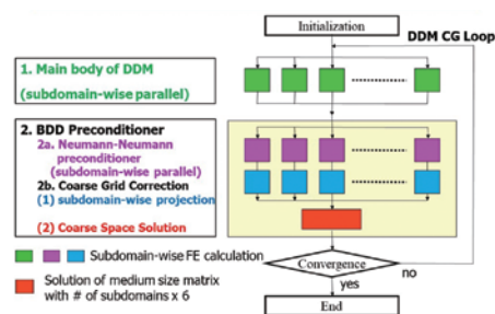
▲図1 ADVENTURE_Solid2のHDDM-BDDソルバーの処理の流れ
