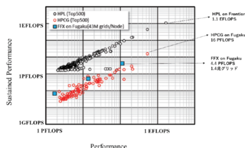
▲図1 Top500におけるHPL、HPCGの性能およびFFXの富岳におけるWeak Scaleベンチマークテスト結果
