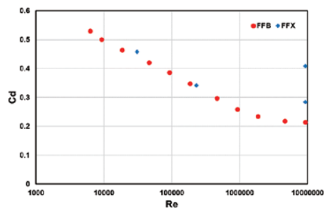
▲図3 車両の抵抗係数のレイノルズ数依存性
